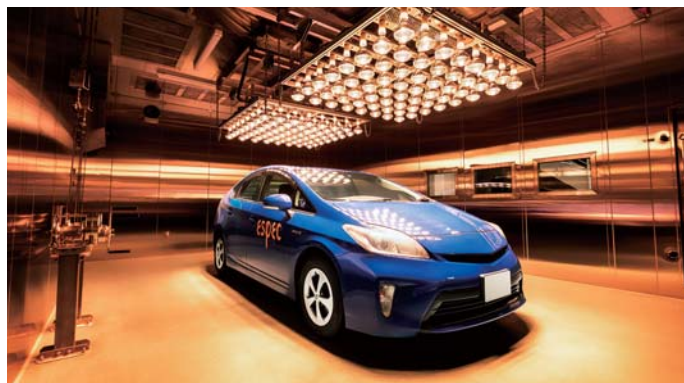
自動車が一台入る実車試験装置
