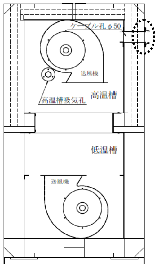
正面図
